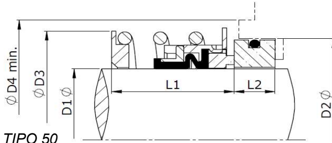
DIMENSIONAL - TIPO 50
